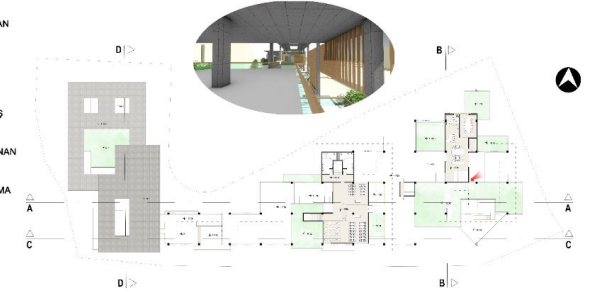
+13.50 KOTU PLANI 1/200
