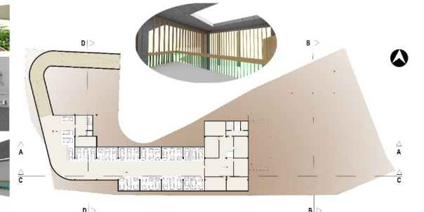
-4.00 KOTU PLANI 1/200
